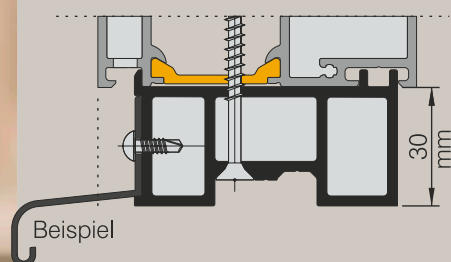
TYP ST 105 Separates Fenster mit D/DK Flügel und Fensterbank- Anschlußprofil 30 mm (ohne Fensterbank)
