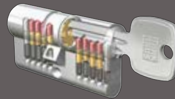
STANDARD - PROFILZYLINDER
