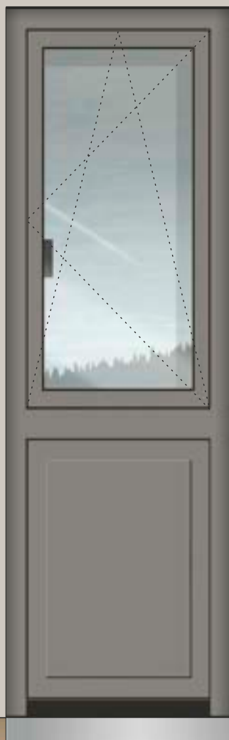
TYP ST 103 Separates Seitenteil mit D/DK Flügel und Paneel unten
